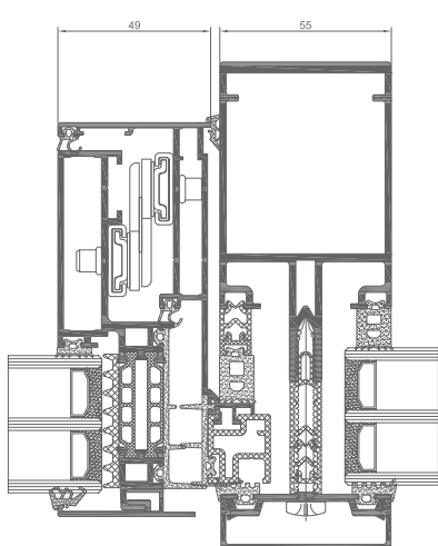
Querschnitt Ausstellfenster MC PW (MC047 + MC143 + MC413 + MC144 + DK053)
