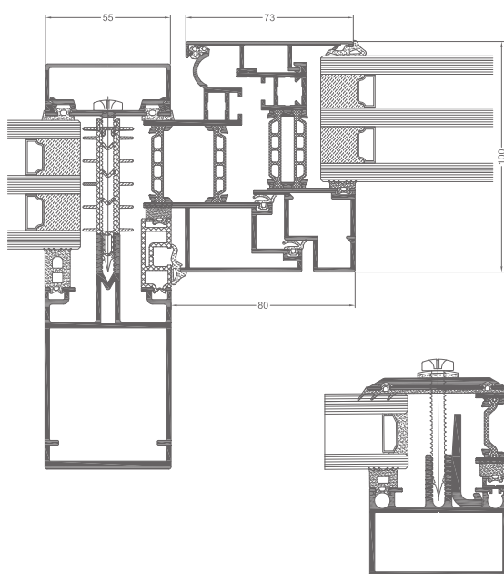
Querschnitt Fenster MC RW, Anschluss des Flügels MC321 an den Pfosten (Öffnung mit Stellantrieb) (MC413 + MC311 + MC321)
