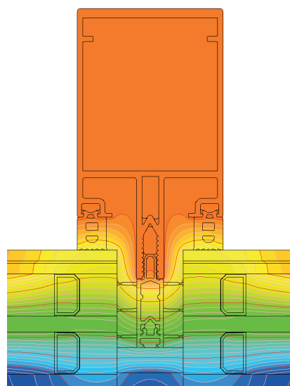
Beispielhafte Isothermenverteilung für das System MC GLASS (MC413)
