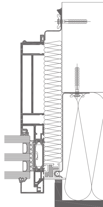
Verbindung des Systems MS an die Baukonstruktion (MS102)
